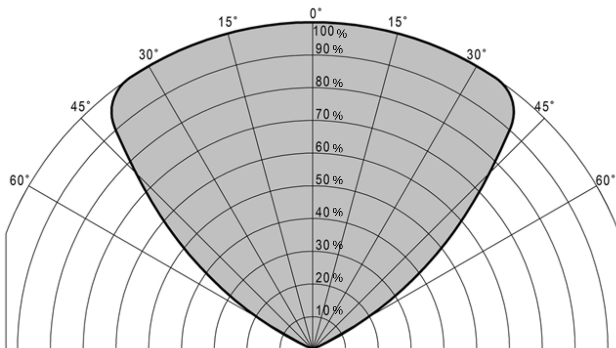
Рисунок 4 – Зависимость дальности обнаружения очага пламени от его углового положения в поле зрения ИПП, в процентах от максимального значения
